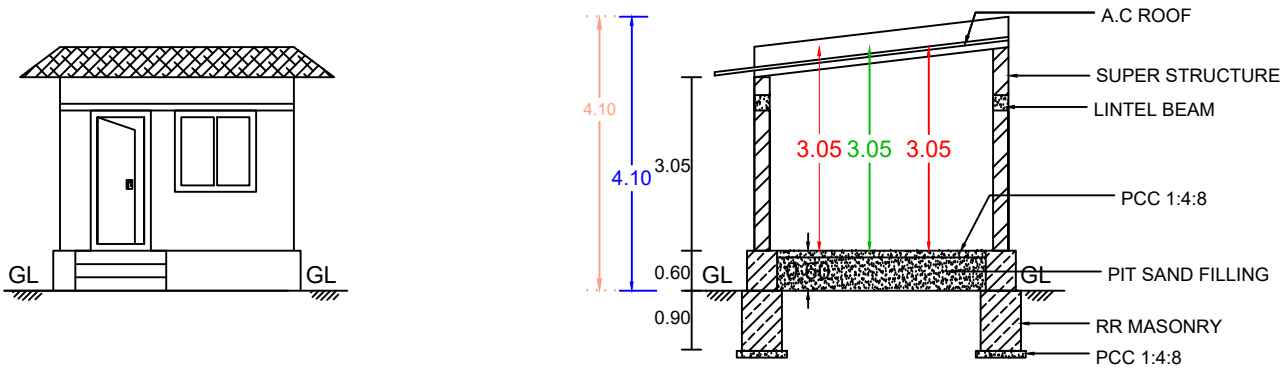
ELEVATION
