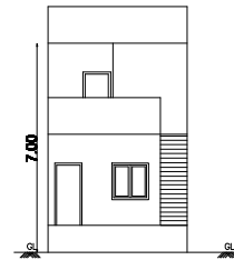
ELEVATION-A
