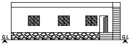
ELEVATION
