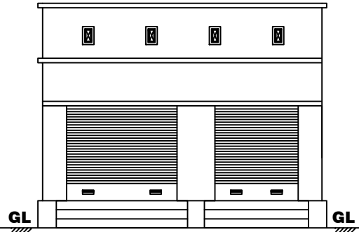
ELEVATION
