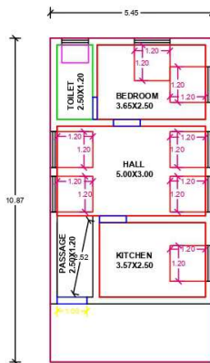
PRO.F.F.PLAN
