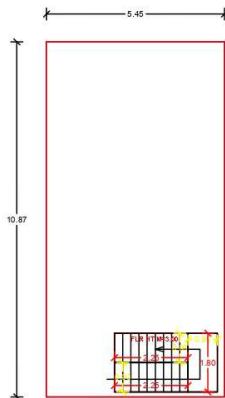
EXG.G.F.PLAN
