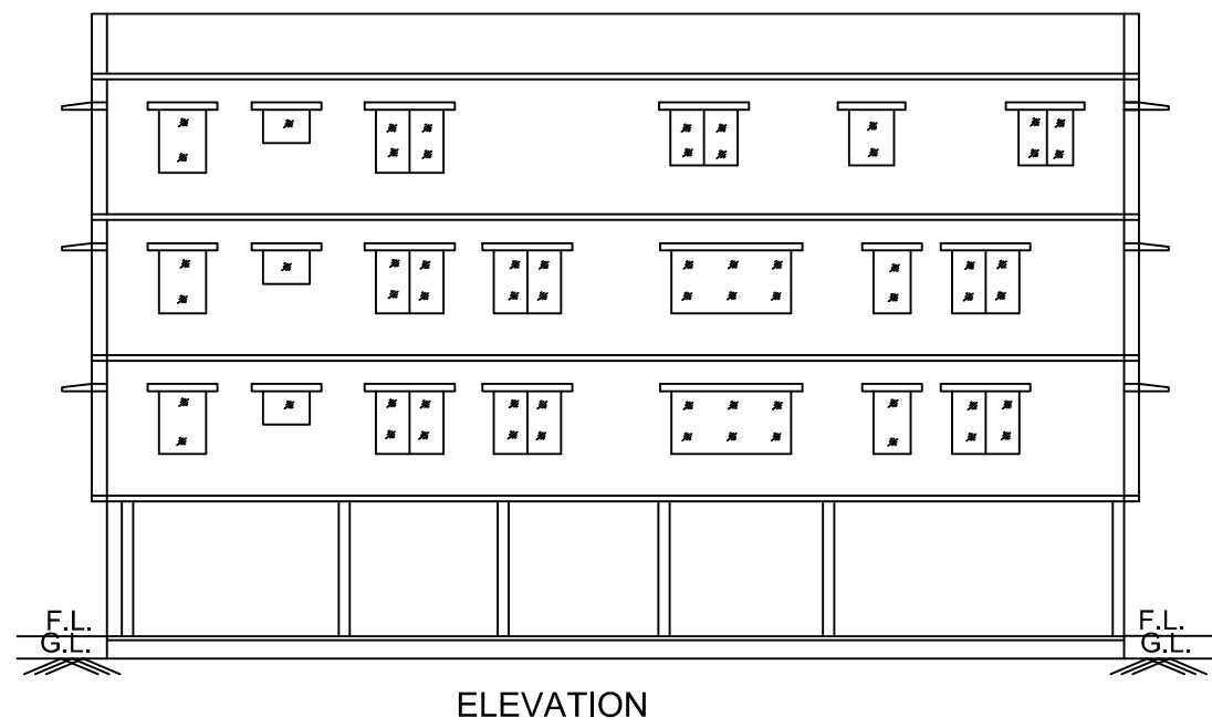
ELEVATION
