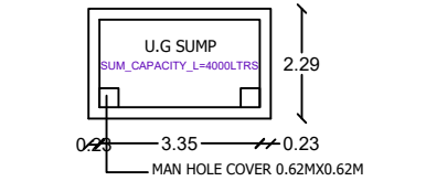
U.G.SUMP
