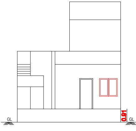
ELEVATION-A
