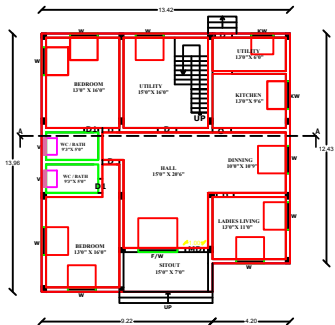
PLAN SCALE : 1:100
