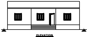
ELEVATION
