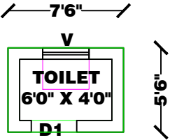
TOILET PLAN
