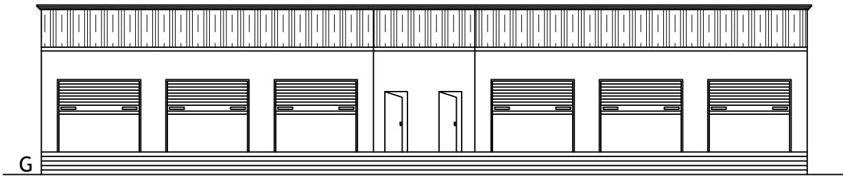
ELEVATION
