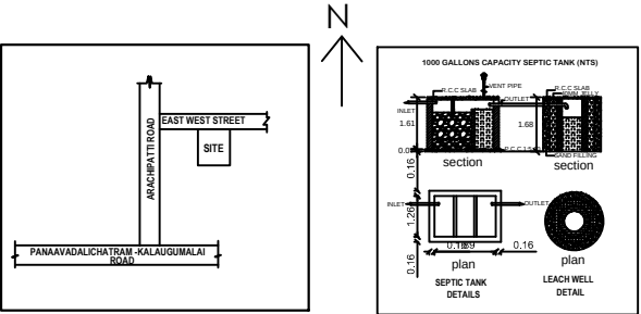
SITEPLAN
