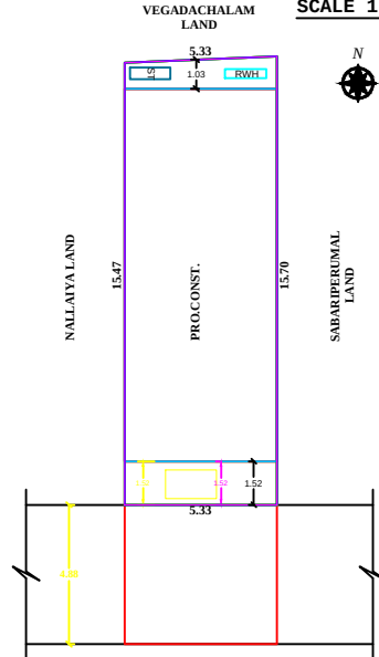
SITE PLAN SCALE 1:100
