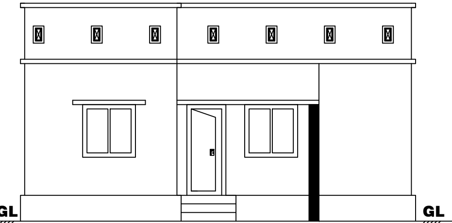
ELEVATION
