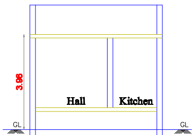
SECTION-A
