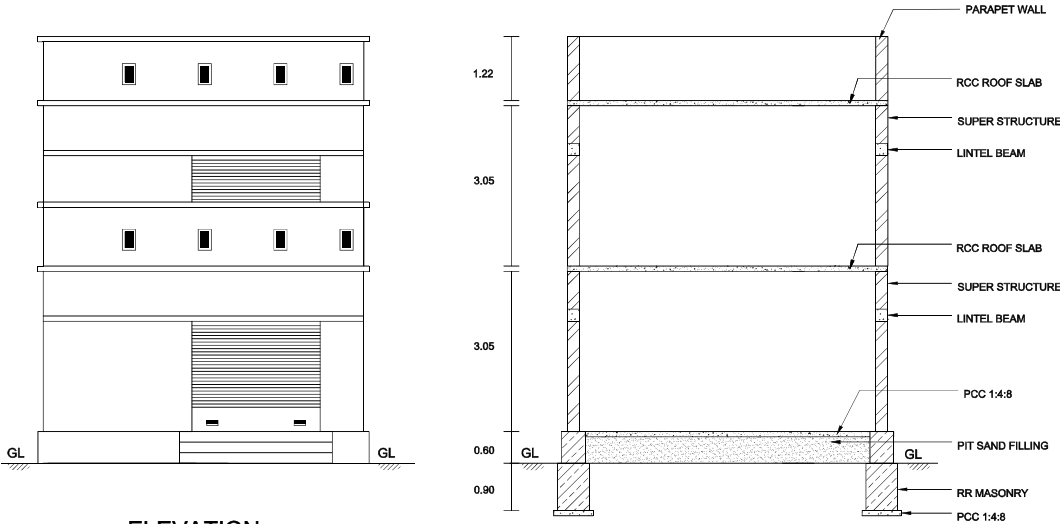
ELEVATION
