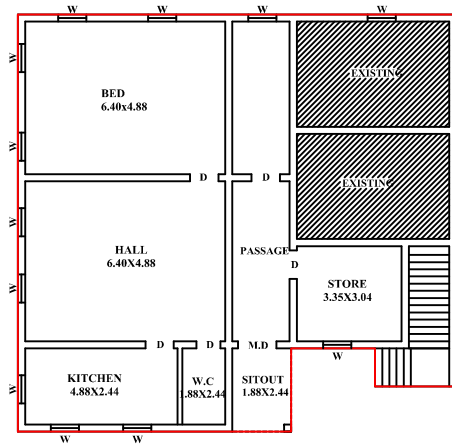
EXISTING G.F.PLAN
