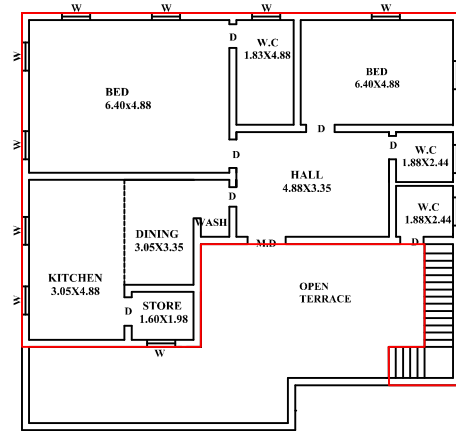
EXISTING F.F.PLAN
