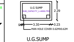
U.G.SUMP
