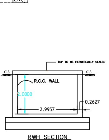
R.W.H. SECTION
