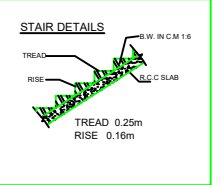
SCALE:- 1:100
