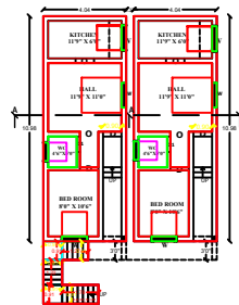
PLAN SCALE : 1:100
