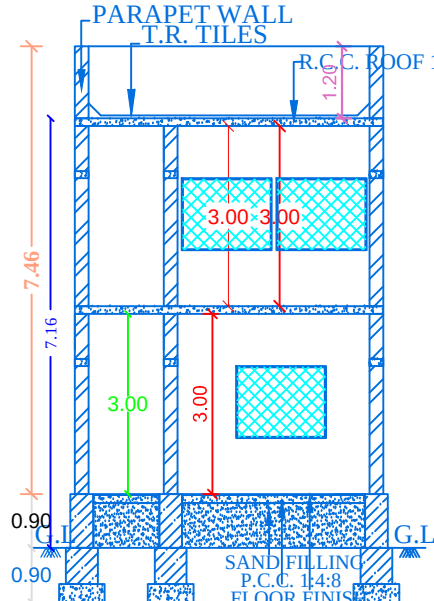
SECTION ON 'AA' 'BB'
