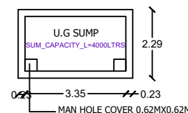
U.G.SUMP
