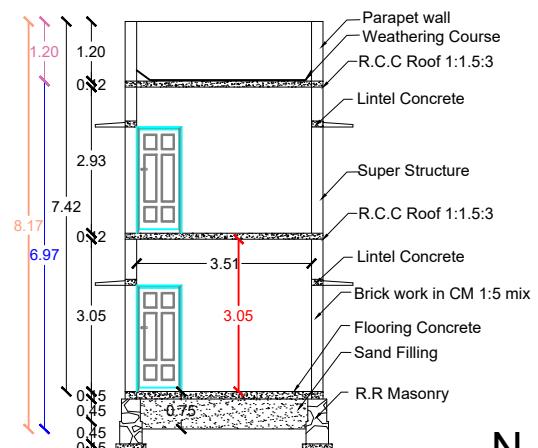
SECTION-E1E1
