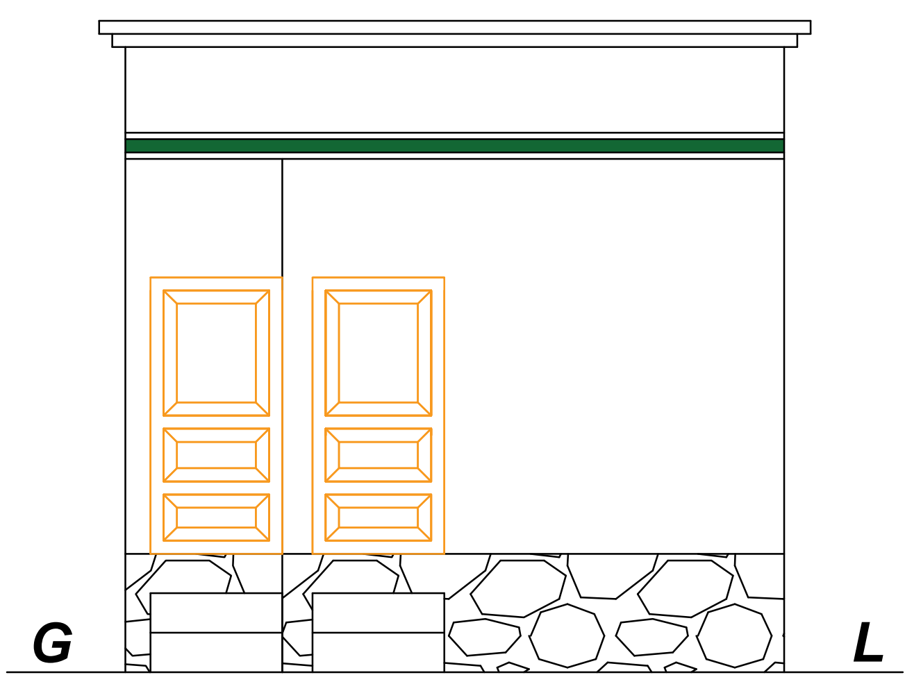
ELEVATION
