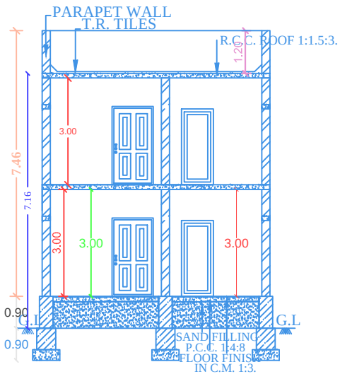
SECTION ON 'AA' 'BB'
