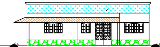
ELEVATION
