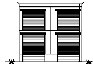
ELEVATION
