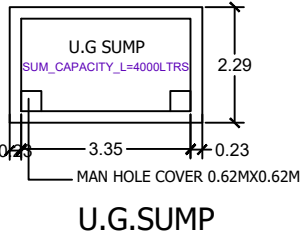
U.G.SUMP
