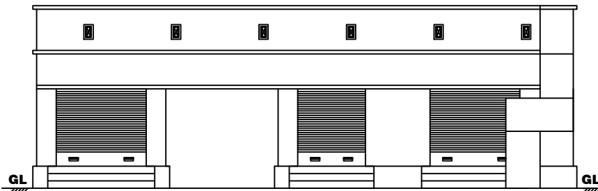
ELEVATION
