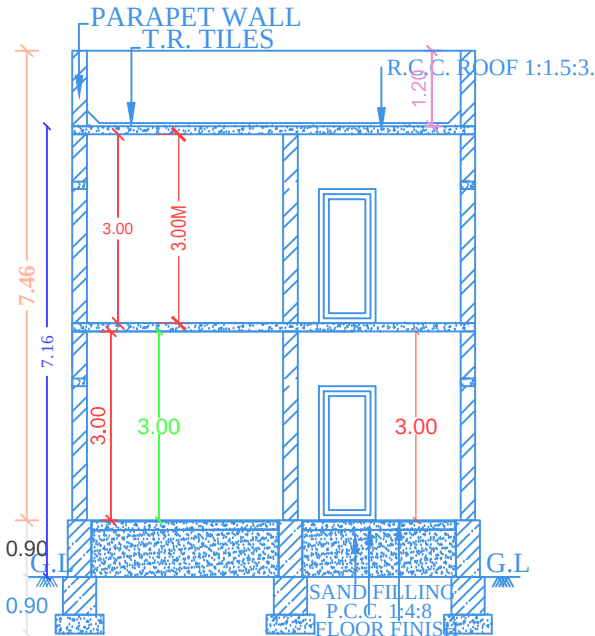
SECTION ON 'AA' 'BB'
