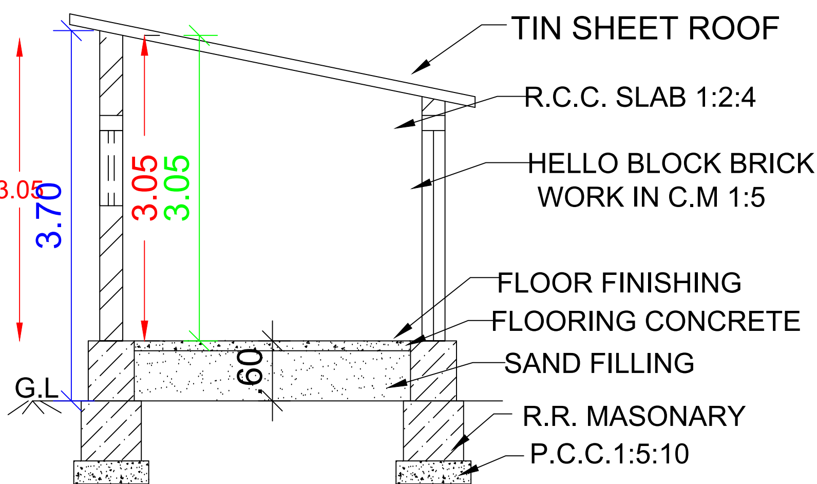
SECTION - AB
