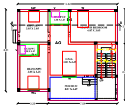
PLAN SCALE : 1:100
