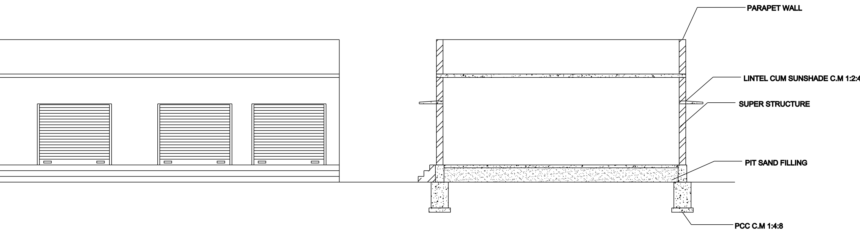
ELEVATION
