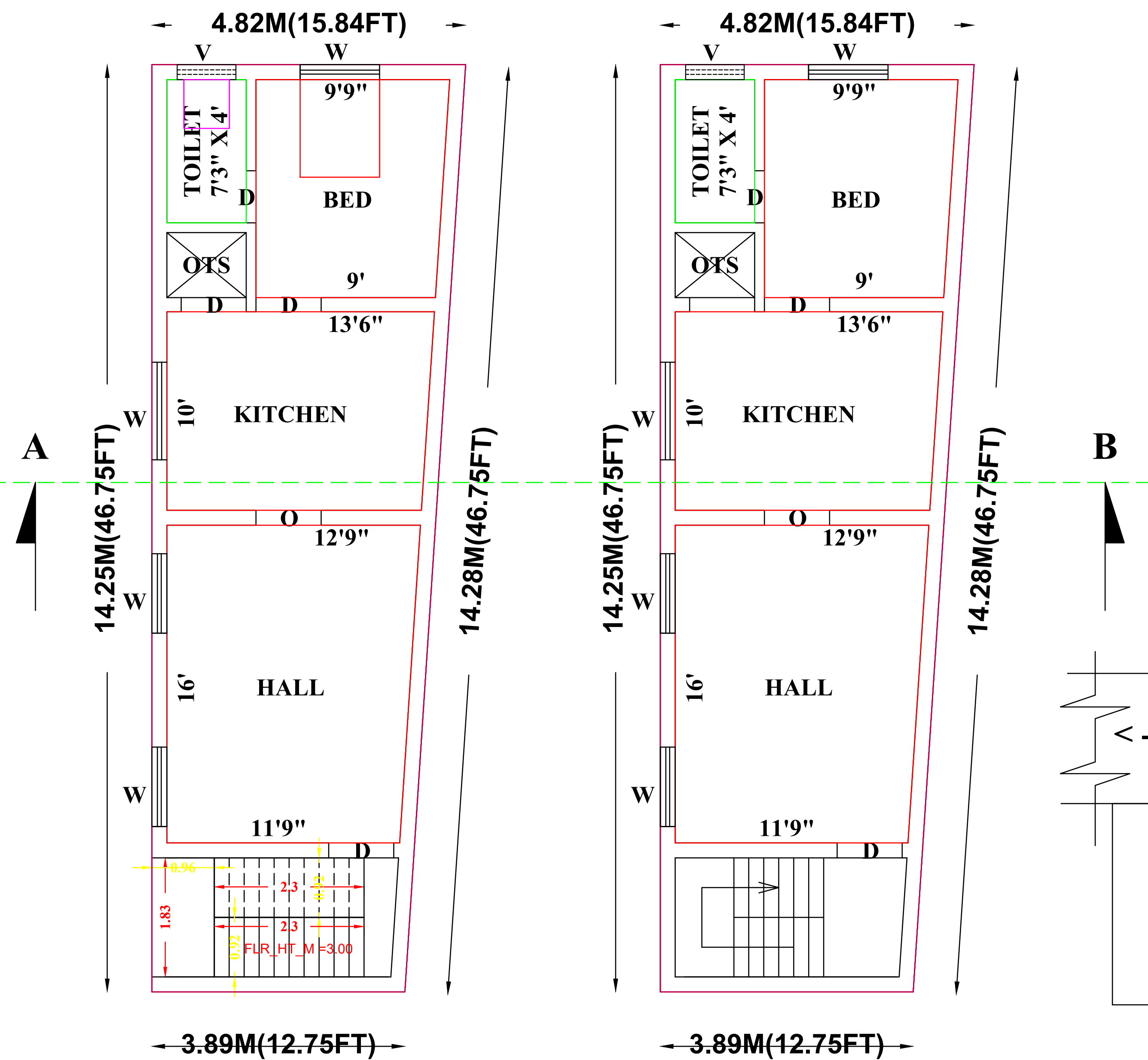
UND FLOOR PLAN
