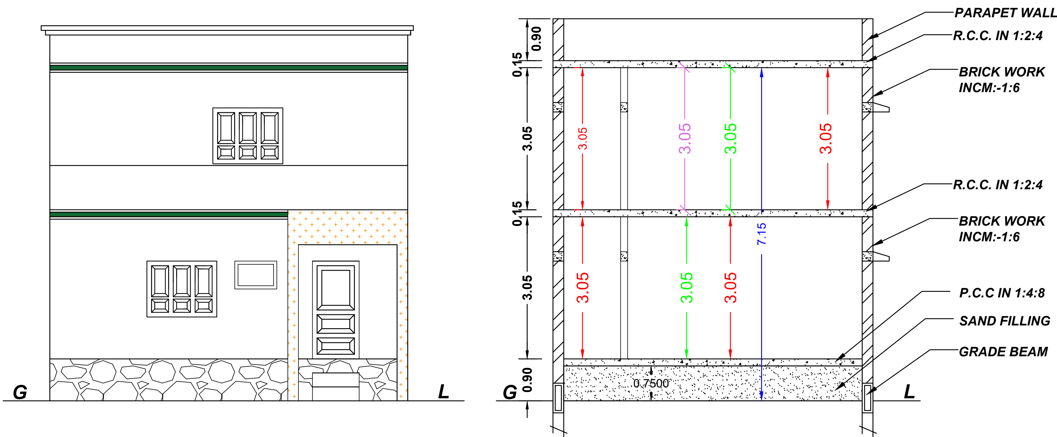
ELEVATION
