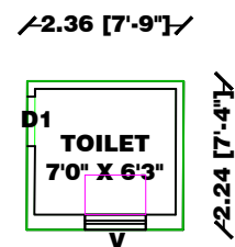
TOILET PLAN
