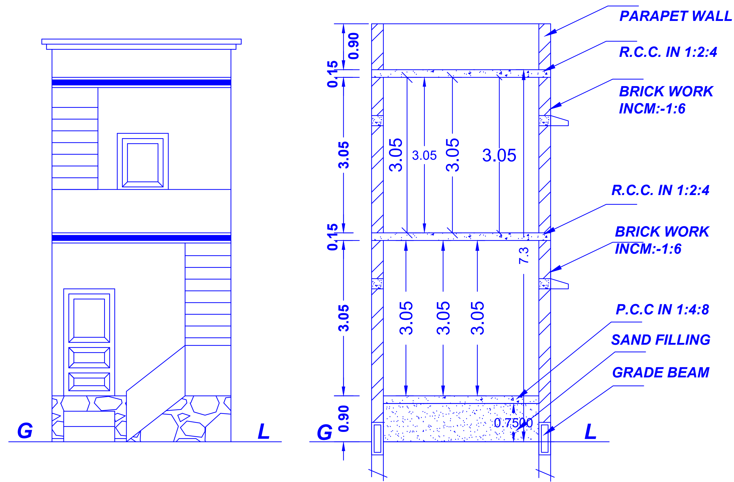
ELEVATION
