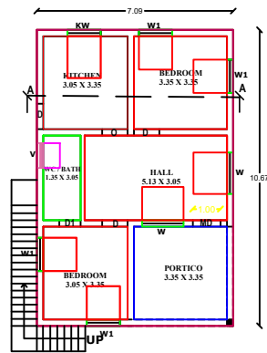
PLAN SCALE : 1:100
