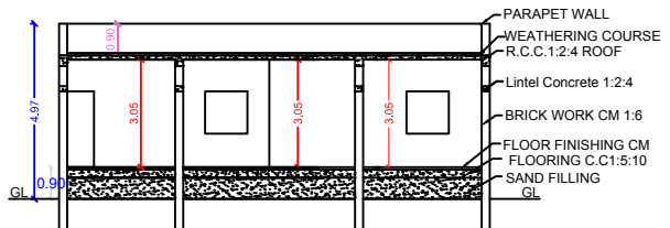
SECTION ON - AZ
