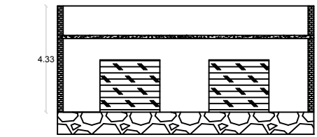
ELEVATION
