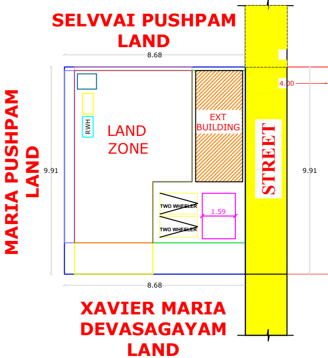
UND FLOOR PLAN
