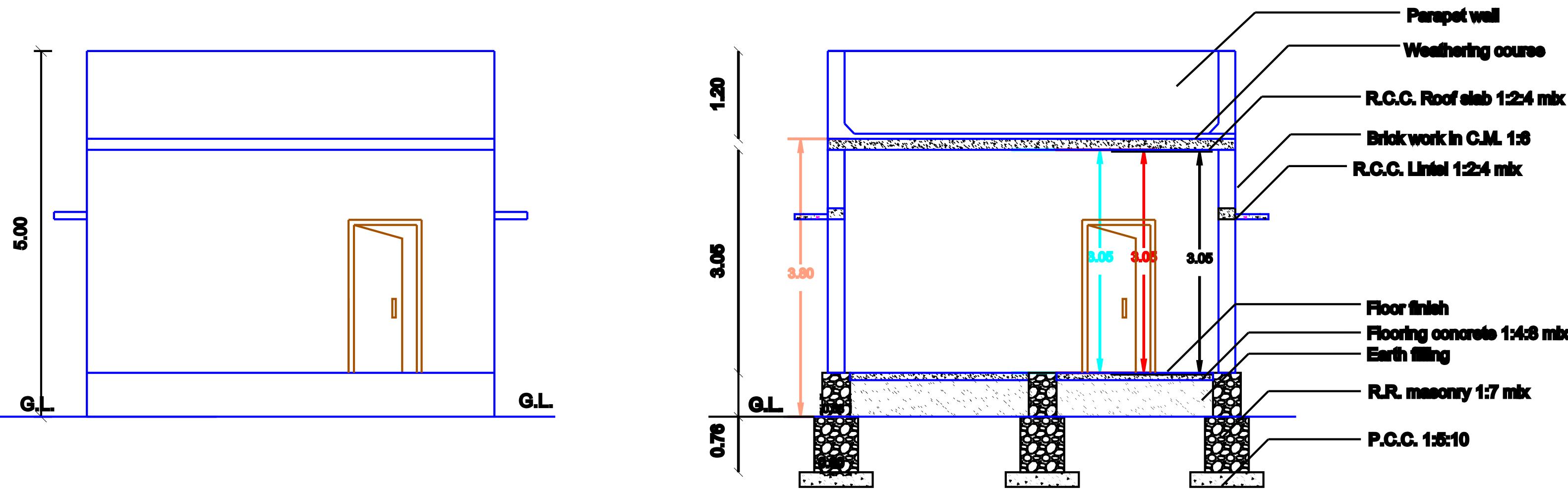
ELEVATION
