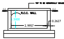
R.W.H. SECTION
