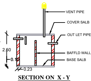
SECTION ON X - Y
