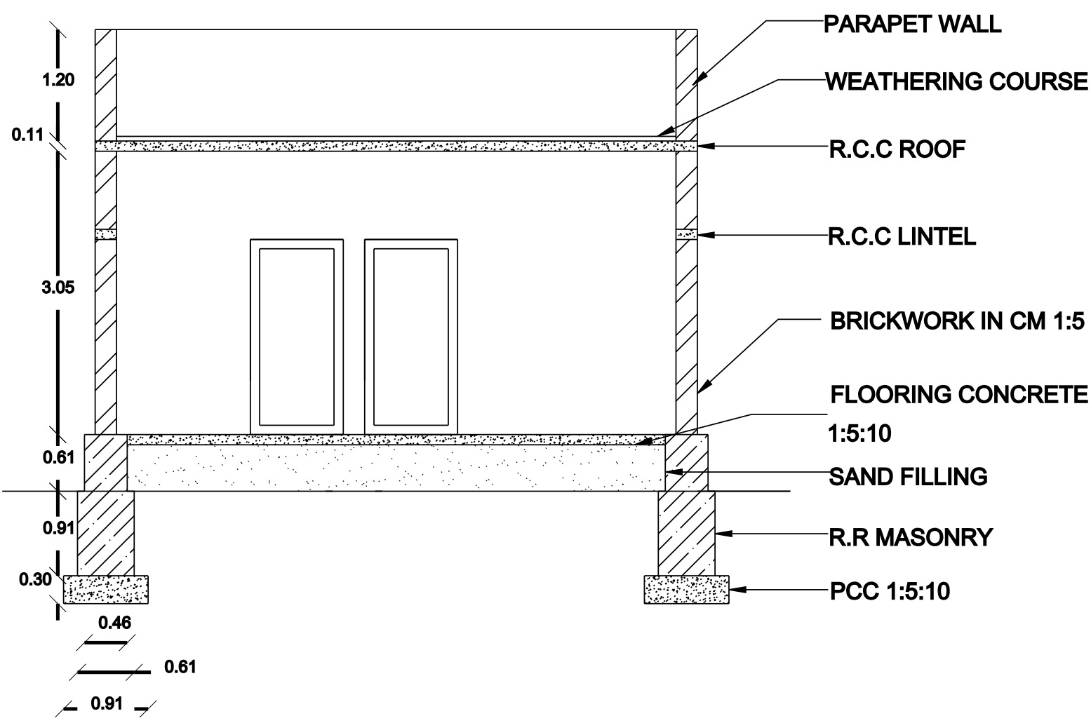
SECTION A-A
