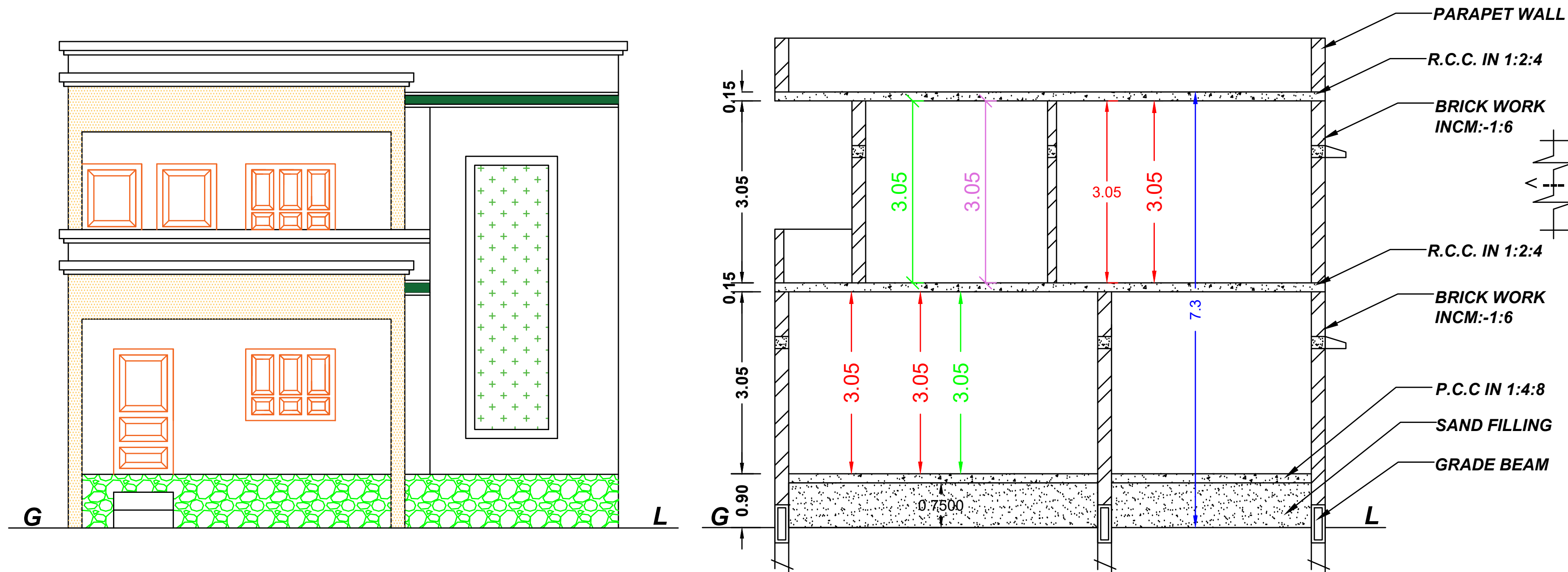
ELEVATION
