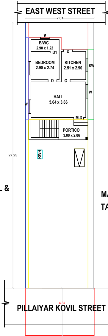
SITE PLAN SCALE 1:100
