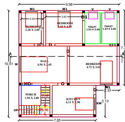
PLAN SCALE : 1:100
