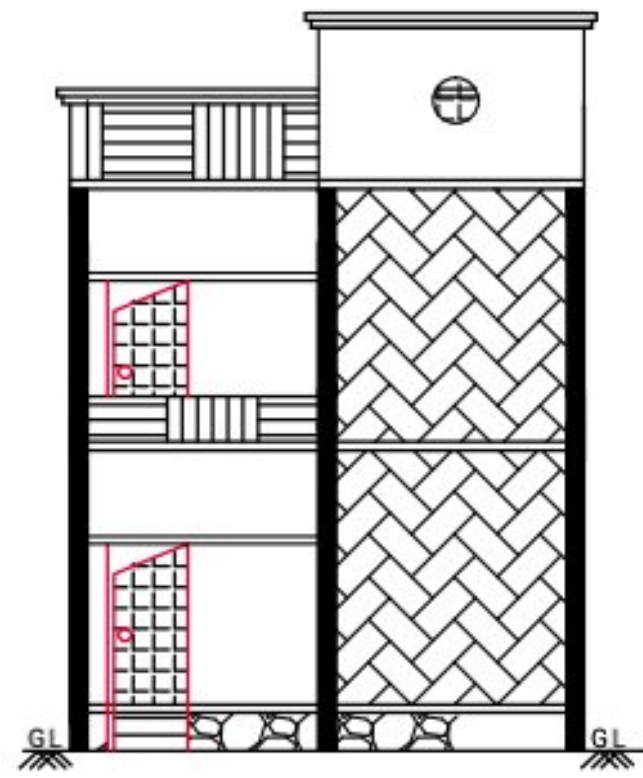
ELEVATION
